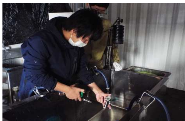
水洗性浸透探傷検査
